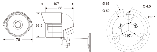
機身尺寸
